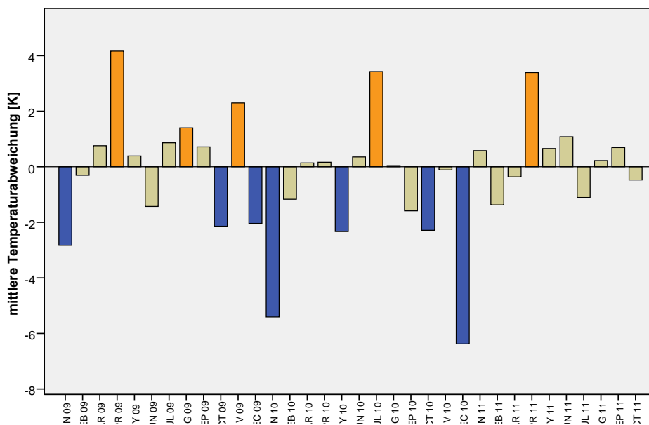
Abweichung der Monatsmittel der Lufttemperatur vom langjährigen Mittel (1951 – 2000) im Zeitraum 2009 bis 2011
